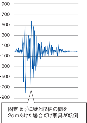
家具の耐震実験 震度7の地震 (関西淡路大震災の揺れ)を再現
