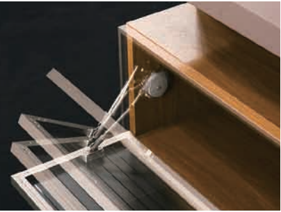
ソフトダウンスティ 標 扉が開きぎる際にゆっくりと静かに開きます。収納されている物にも、接合部にも負担のかからない構造です。
