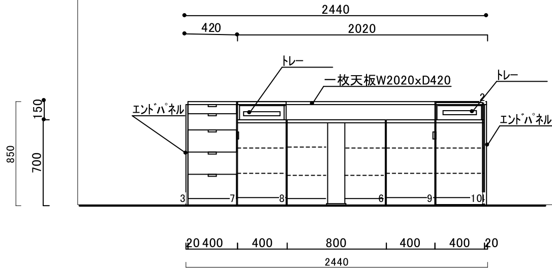
H 正面図 W
